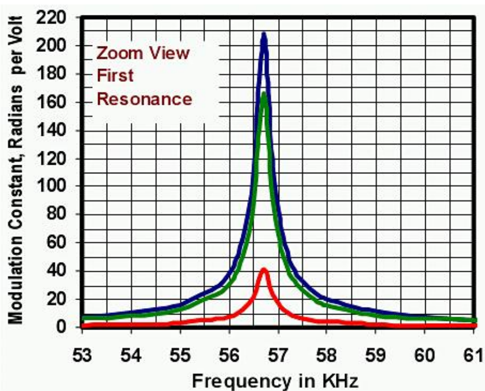
Pizeo-electric 二次谐波振荡响应
