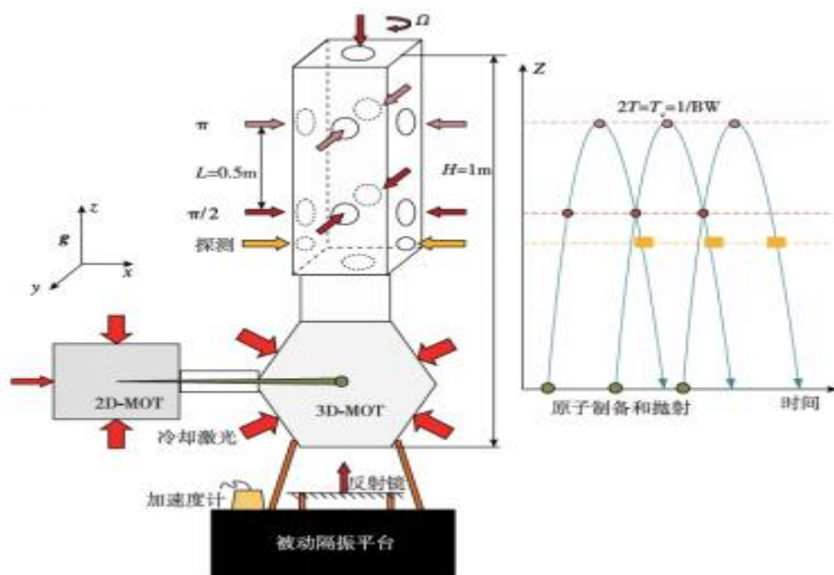
上抛式冷原子干涉重力仪原理框图
