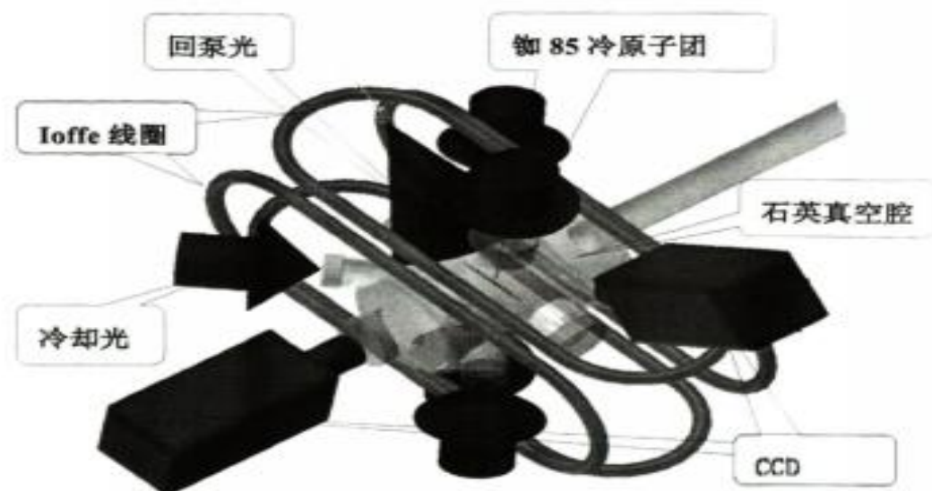
二维磁光阱装置示意图
