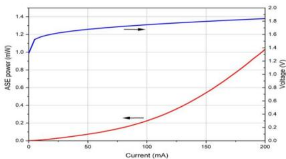
L-I-V 曲线
