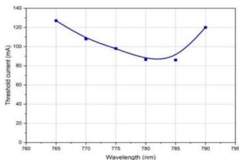
阈值电流
