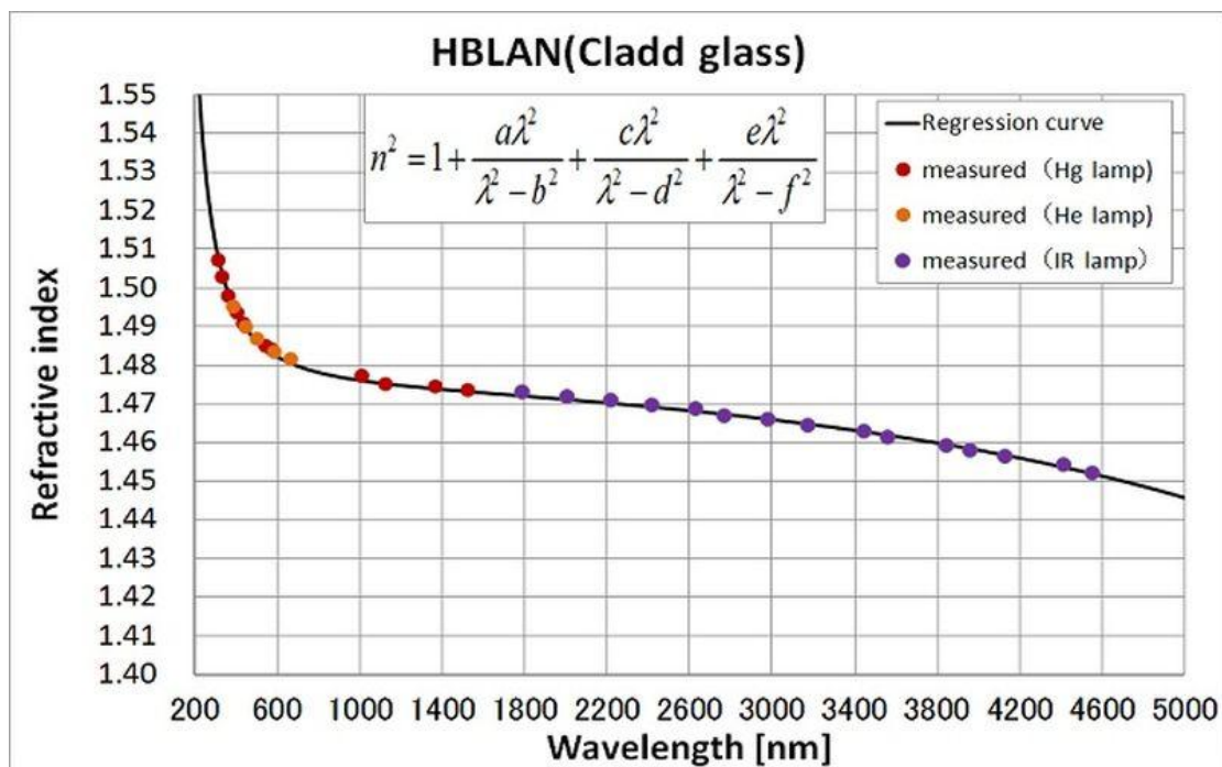
HBLAN 玻璃的折射率 (用于包层, 典型)
