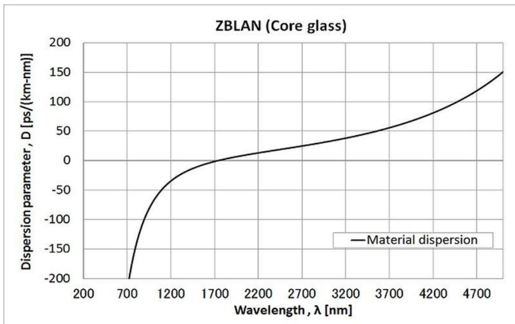
ZBLAN 玻璃的材料分散性（芯，典型）
