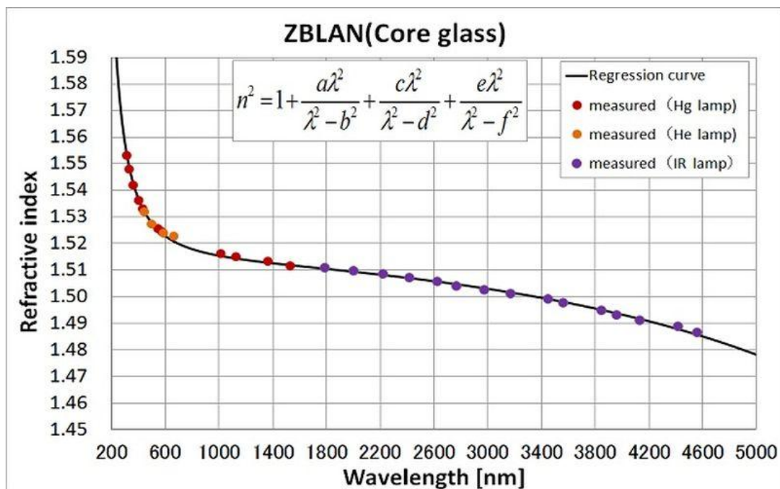
ZBLAN 玻璃的折射率 (芯, 典型)
