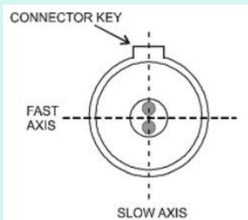
连接器与熊猫光纤对齐:
