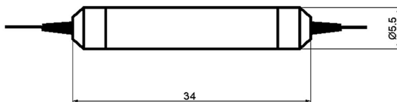
标准尺寸光纤隔离器
