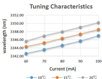
波长调谐曲线
