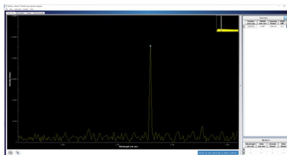
光谱图 (15°C、90mA)
