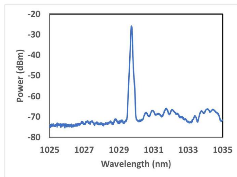
Fig. 4. OEPLS-PS-100-NL MOPA module spectrum
