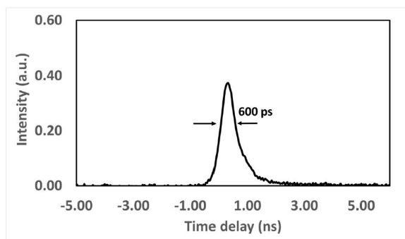
Fig. 5. Pulse width
