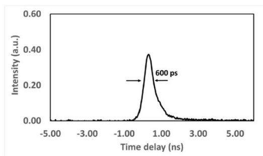
Fig. 5. Pulse width
