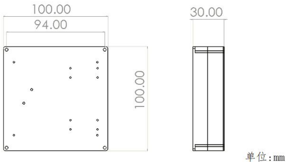
模块尺寸
