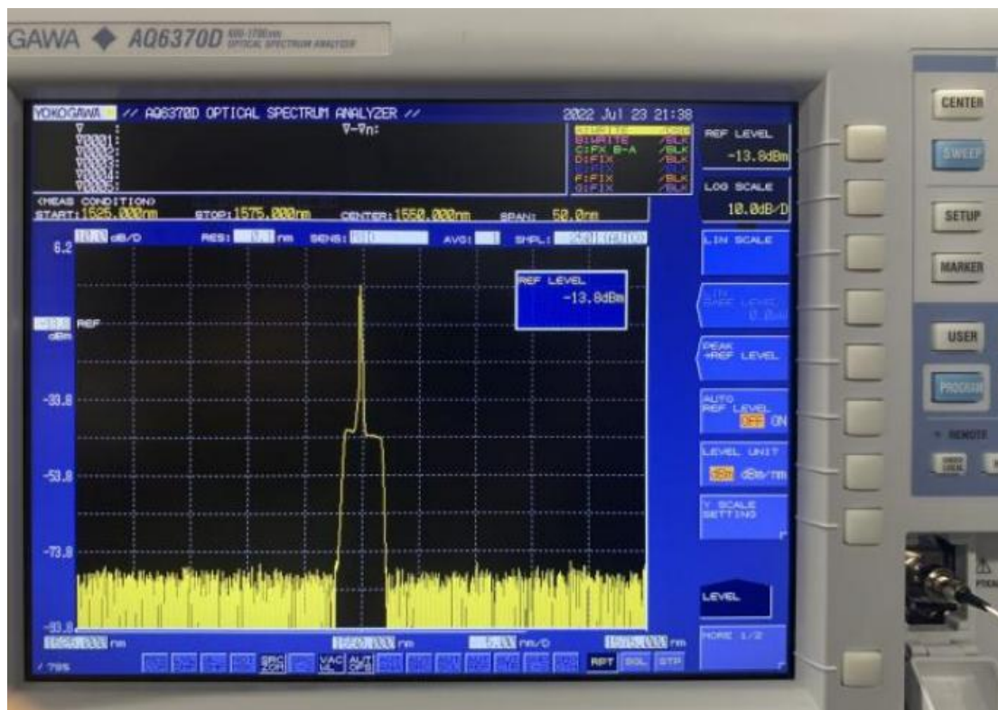
光谱测试@10kHz,3ns,100 \mu J
