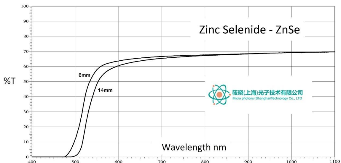
透射曲线图
