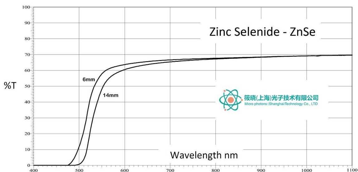
透射曲线图
