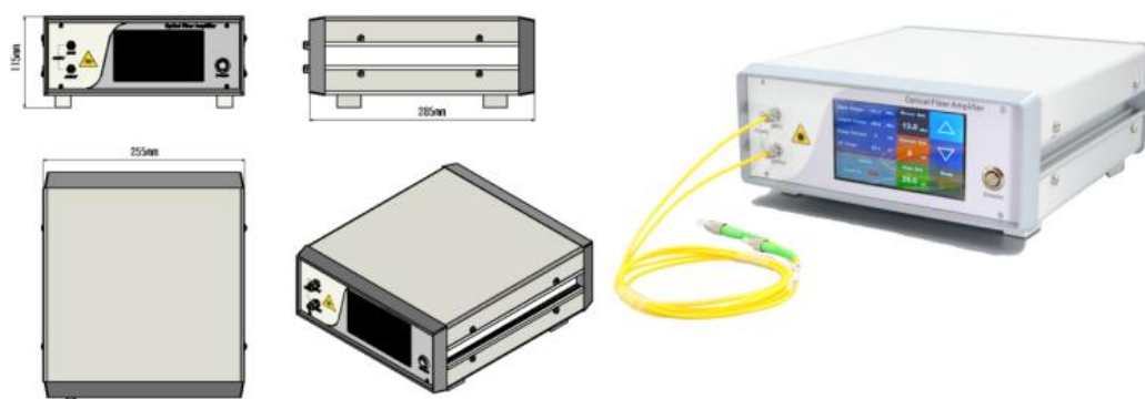
台式实物及尺寸
