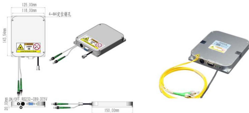
M20 模块式实物及尺寸
