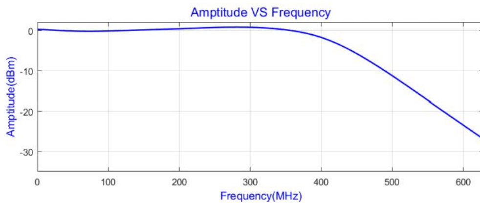
400MHz带宽曲线
