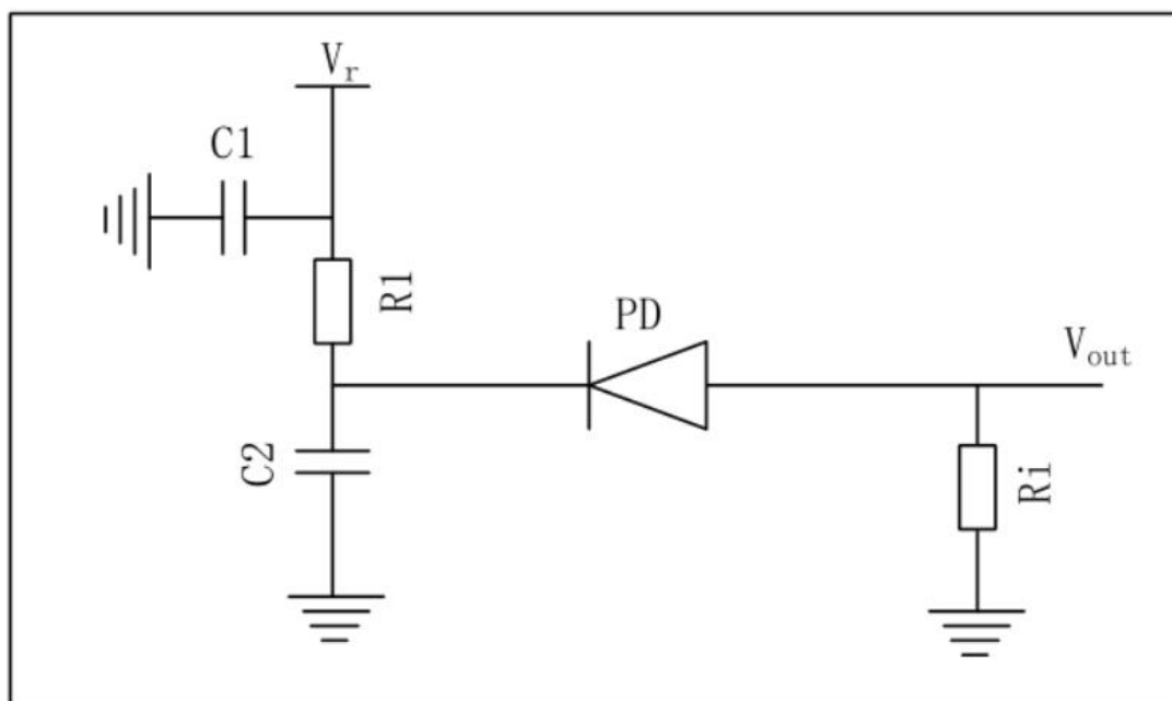
图 6 应用电路图
