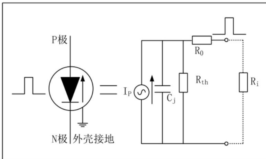
图 5 等效电路图
