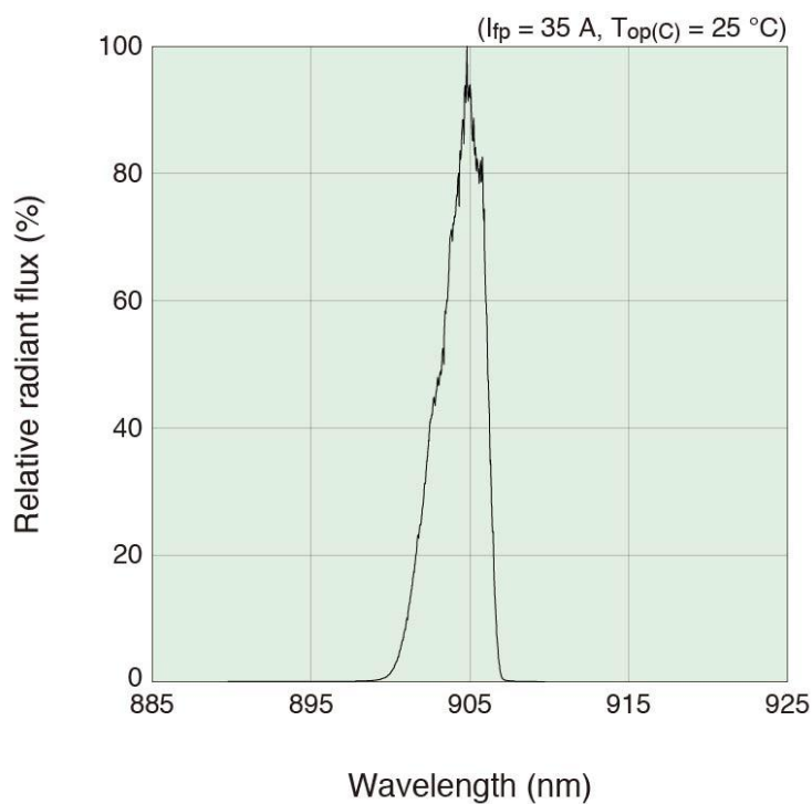
典型发射光谱
