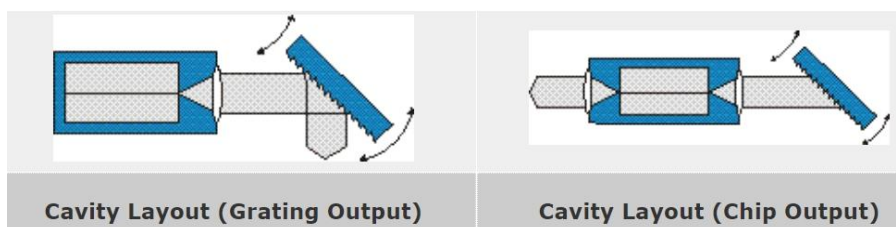
手动可调谐 Littrow 激光系统 - Lynx S3 光栅输出及芯片输出示意图
