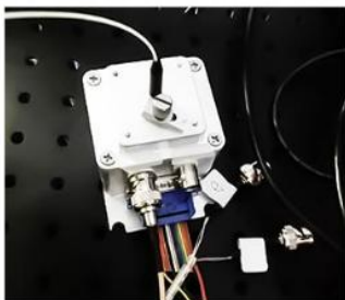
VCSEL激光器测量底座
