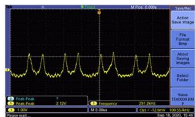
加载5V电压，100KHz频率波形
