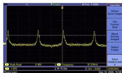
加载5V电压，20KHz频率波形
