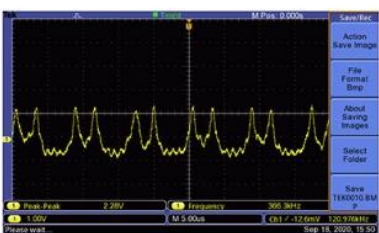
加载5V电压，120KHz频率波形
