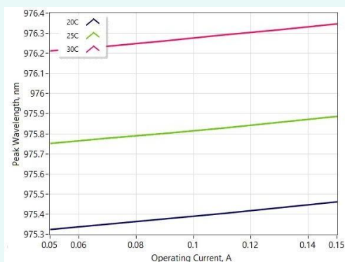
电流峰值波长调谐
