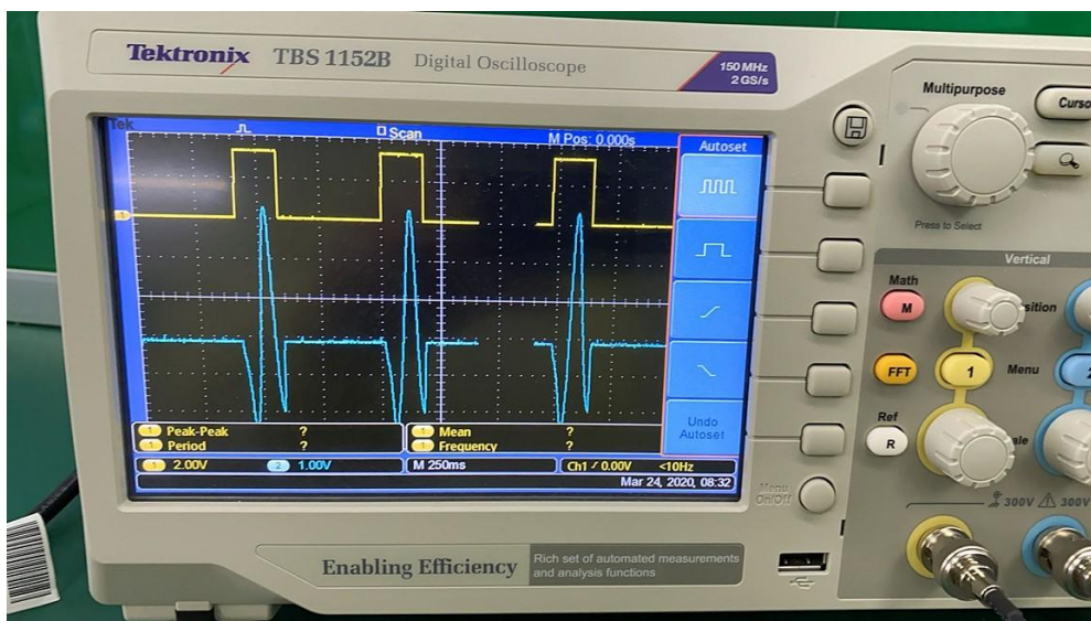
调制信号线性度测试 (示波器电压信号效果图)
