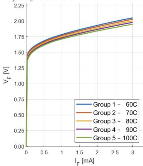
正向电流 1) 2) V_F = f(I_F) ; DC = 100 %
