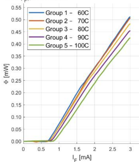
光输出功率 1) 2) \Phi = f(I_F) ; DC = 100 %
