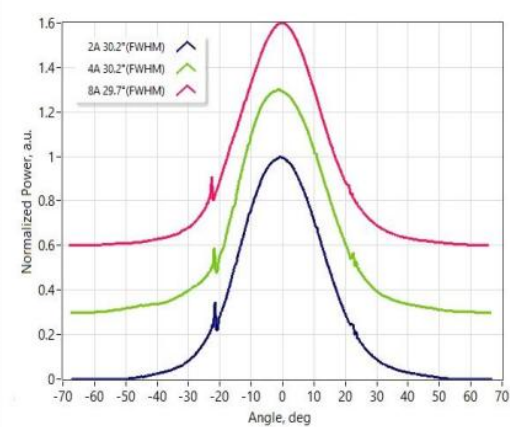
快轴远场
