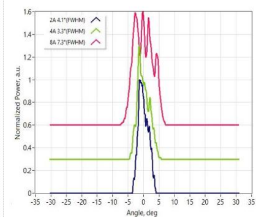
慢轴远场
